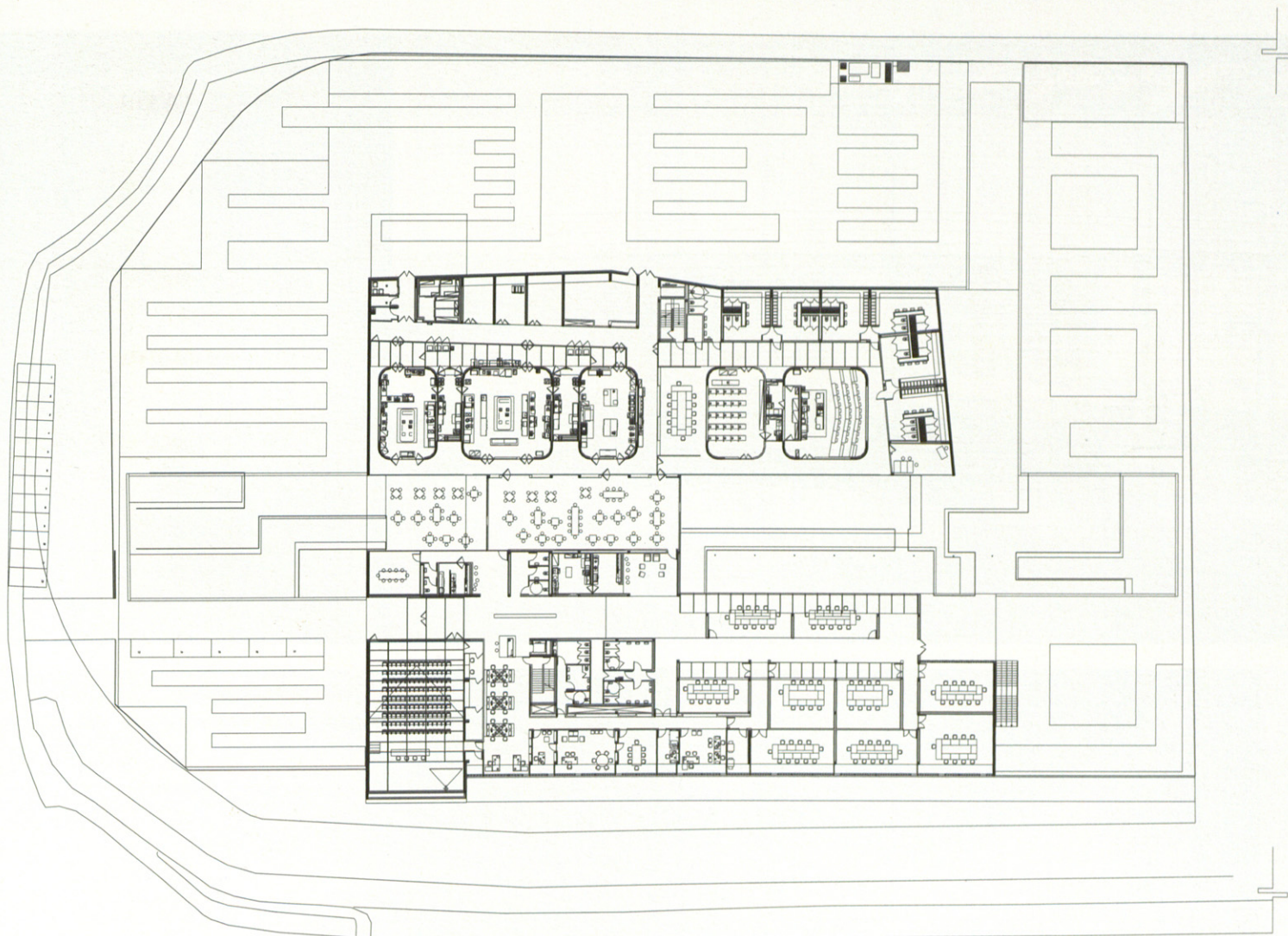
PLANTA BAJA EN LA PÁGINA ANTERIOR, SECCIÓN LONGITUDINAL EN LA PÁGINA SIGUIENTE, SECCIÓN TRANSVERSAL Y ALZADO NORTE
